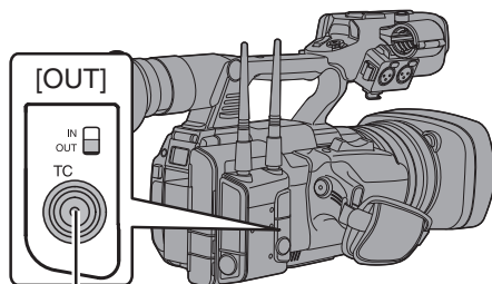
Dispositif principal
